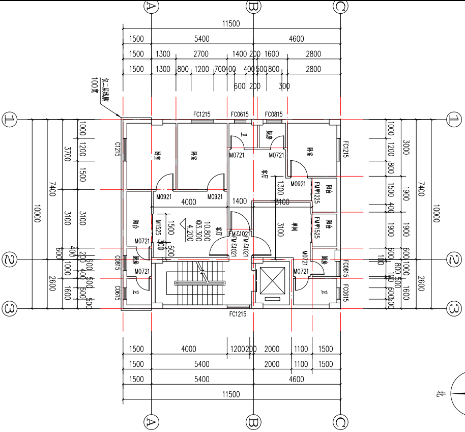
二至四层平面图 1:100
