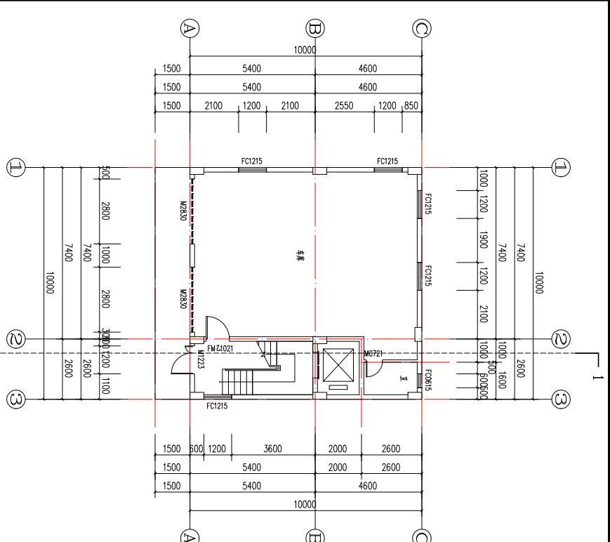
首层平面图 1:100
