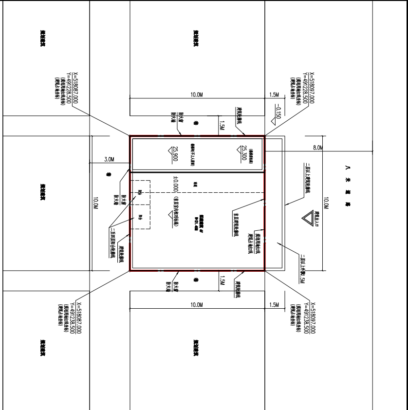
总平面布置图 1:100 注：本项目总用地面积为100㎡，总建筑面积为702㎡。
