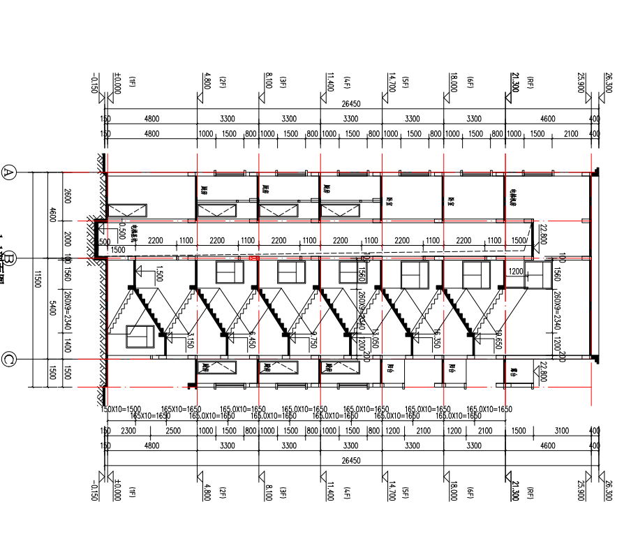
1-1剖面图 1:100
