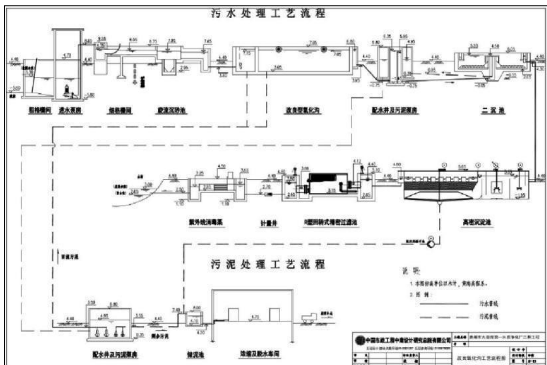
图 4-2 大亚湾第一水质净化厂(二期)处理工艺流程图
