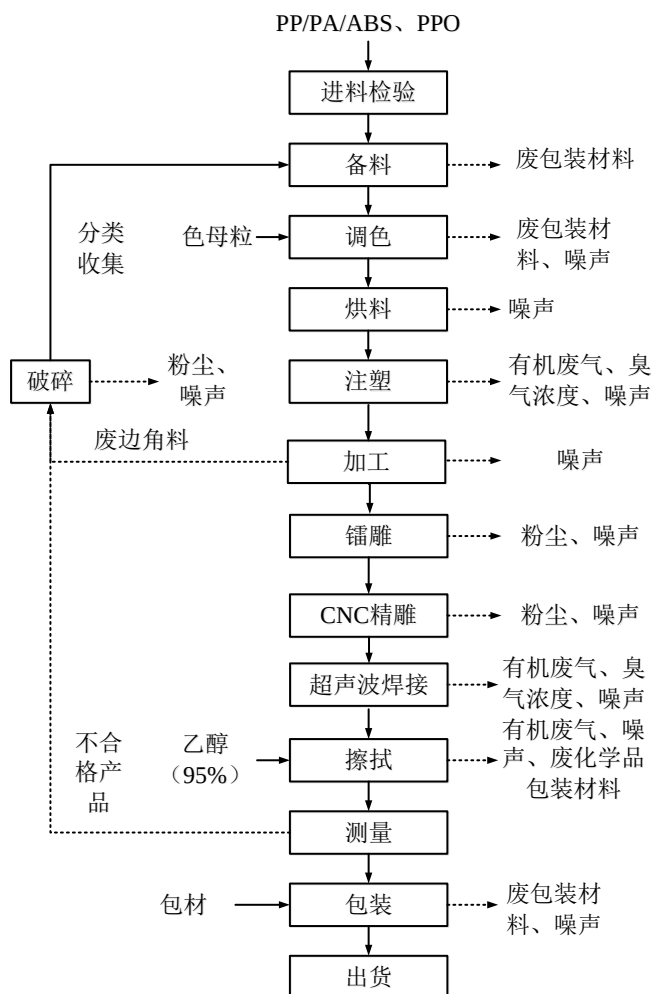
图2-2项目迁建后生产工艺流程图
