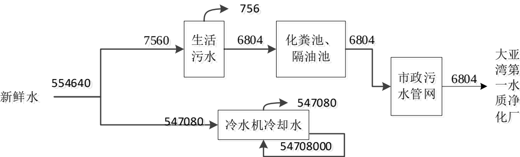
图 2-1 项目迁建后水平衡图（单位：m³/a）
