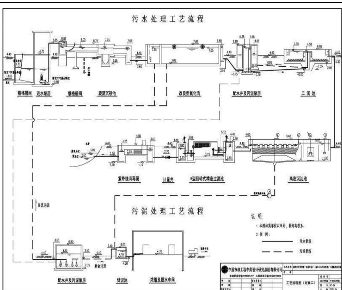
图 4-1 大亚湾第一水质净化厂(一期)处理工艺流程图
