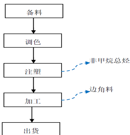
图2-3现有项目生产工艺流程及产污环节图
