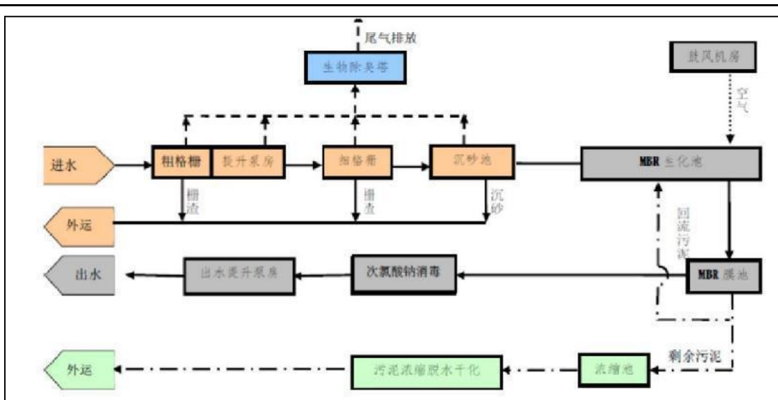
图 4-3 大亚湾第一水质净化厂（三期）处理工艺流程图
