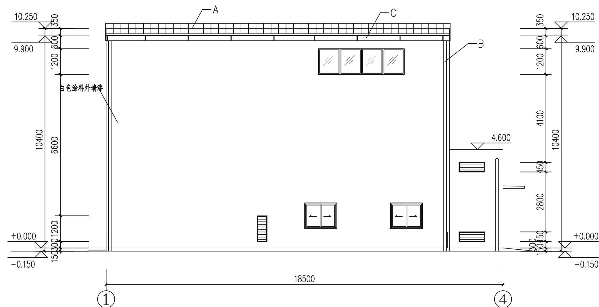
①~④轴立面图
