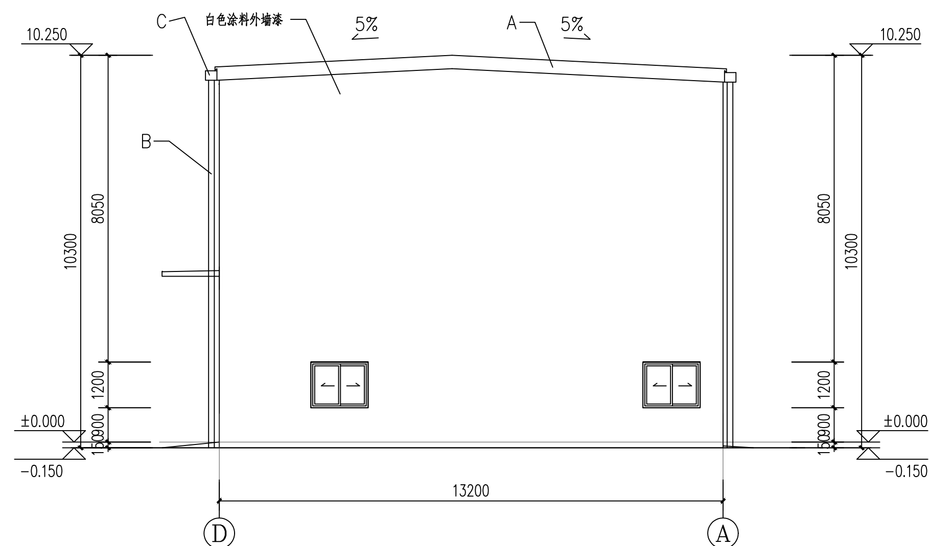
⑩~①轴立面图
