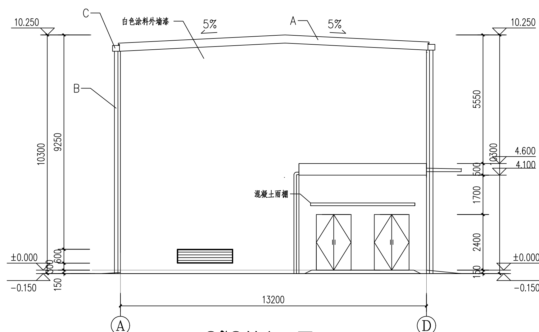
①~⑩轴立面图
