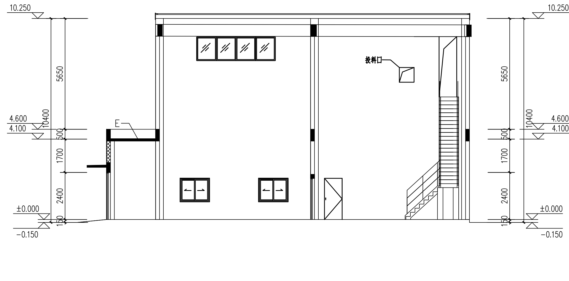
1-1 剖面图
