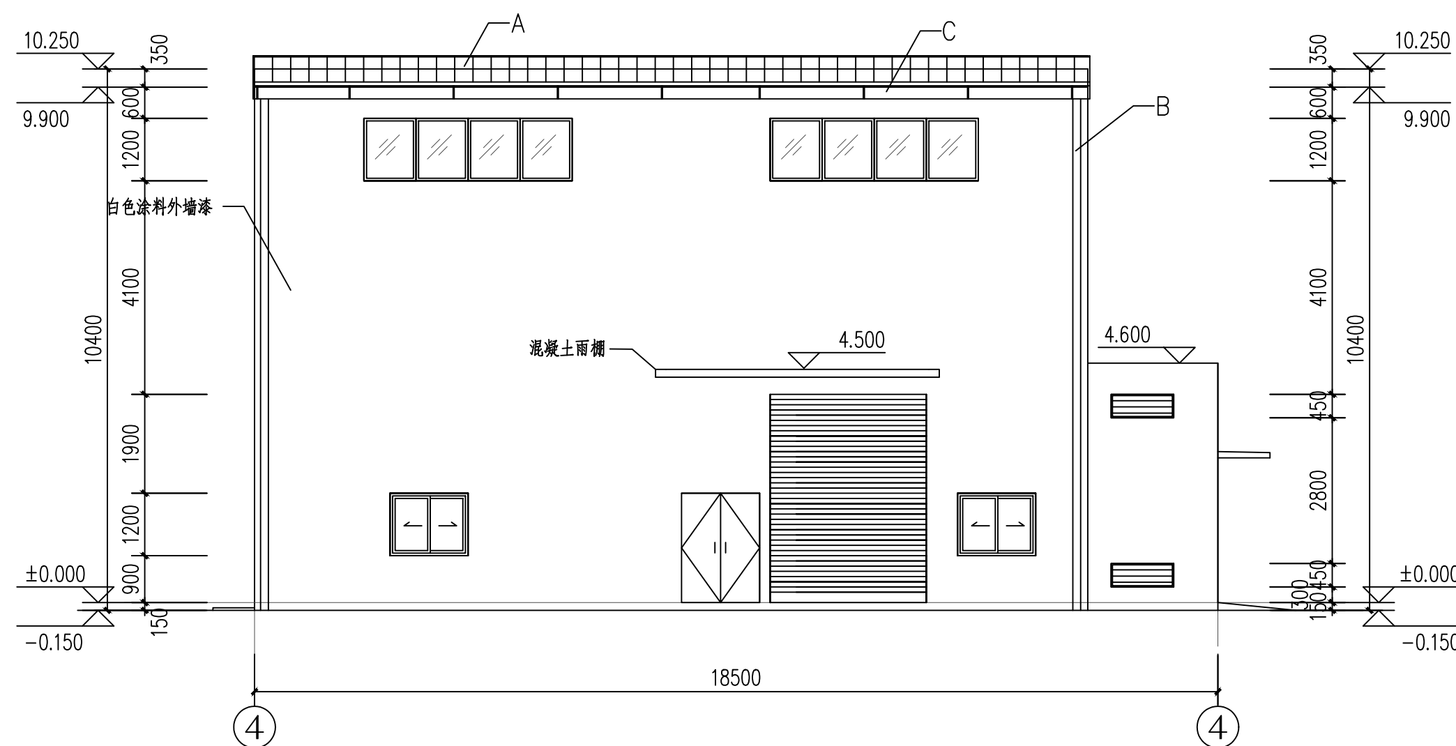
④~①轴立面图
