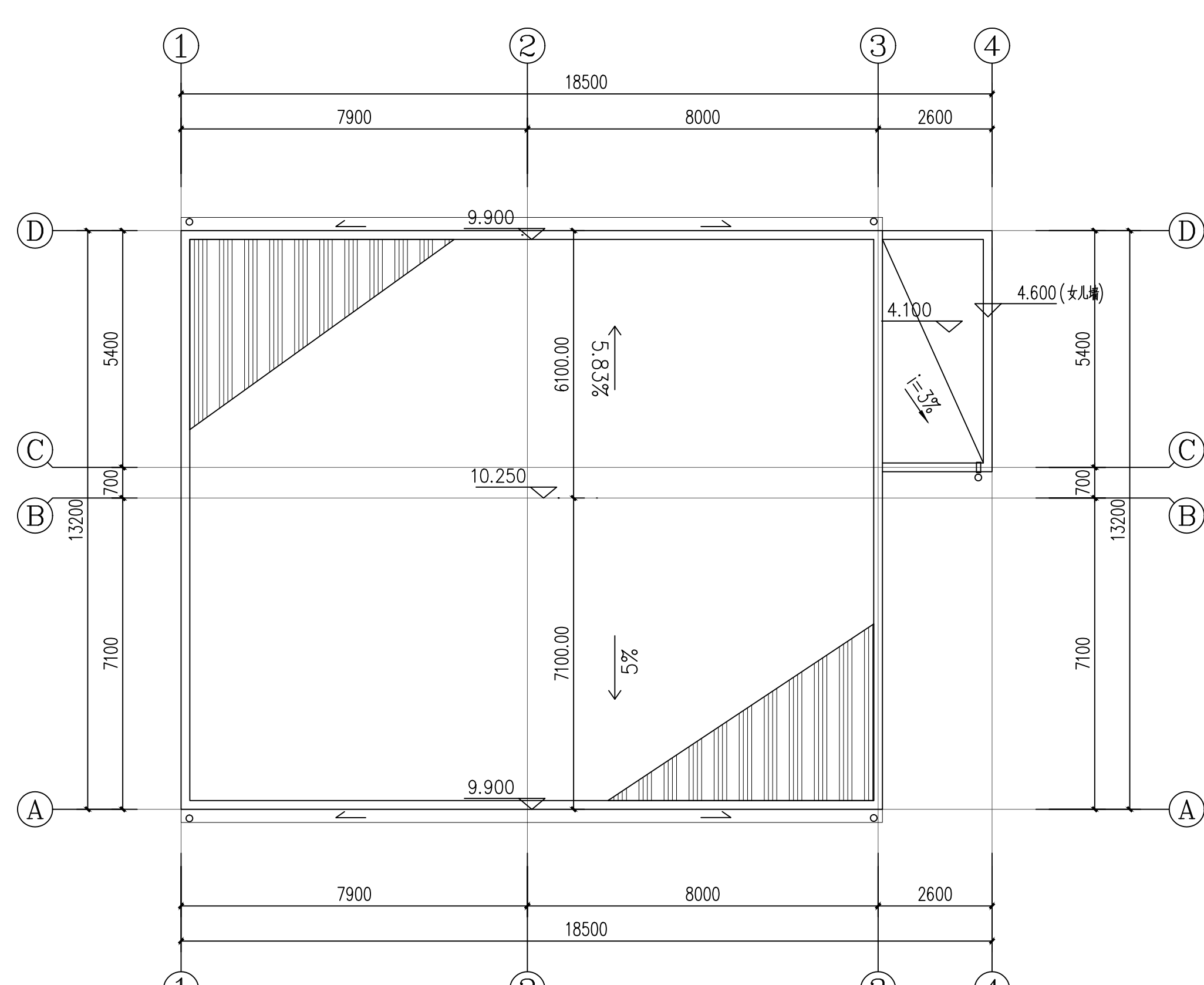
屋面平面图
