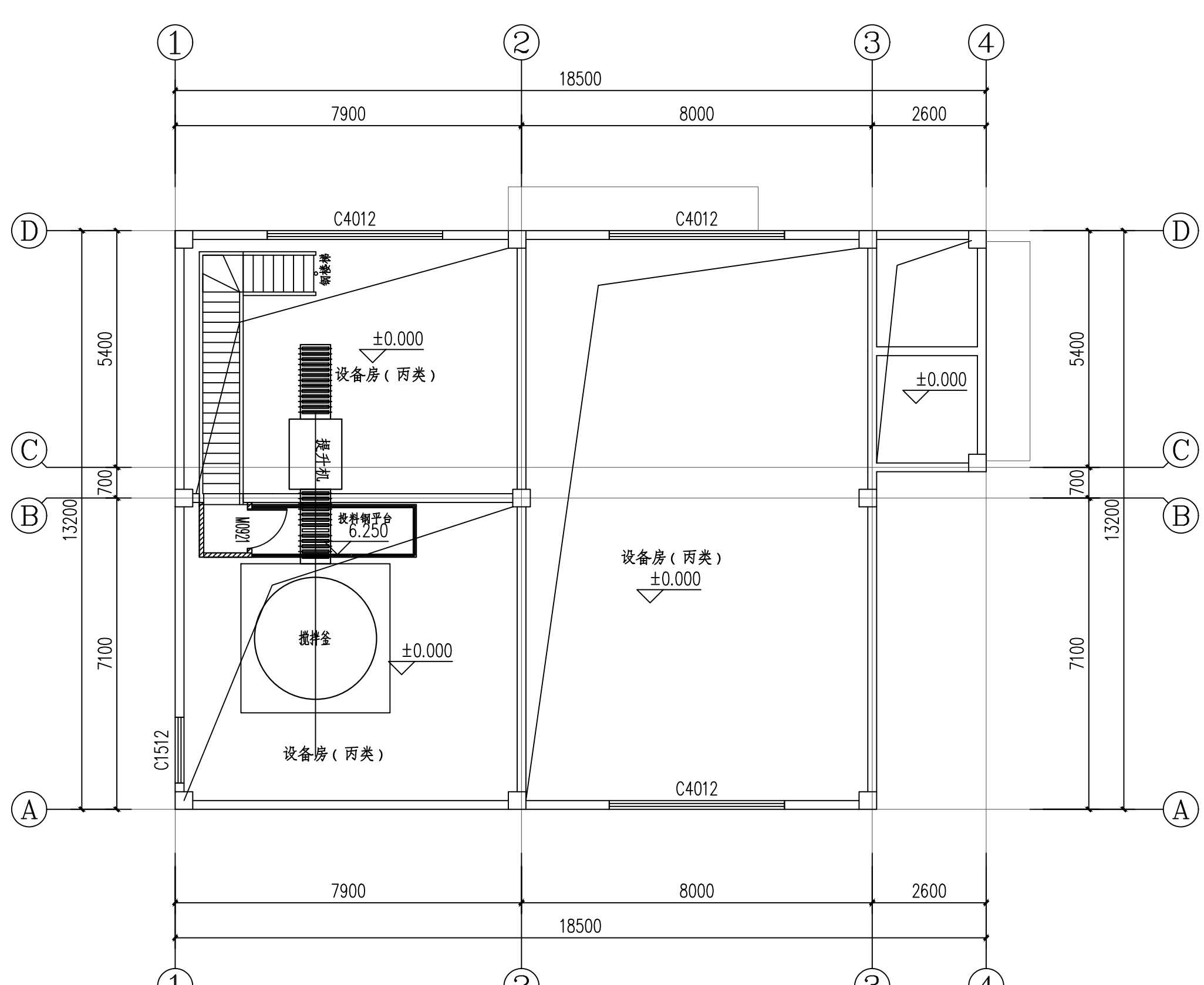
5.000m标高平面图
