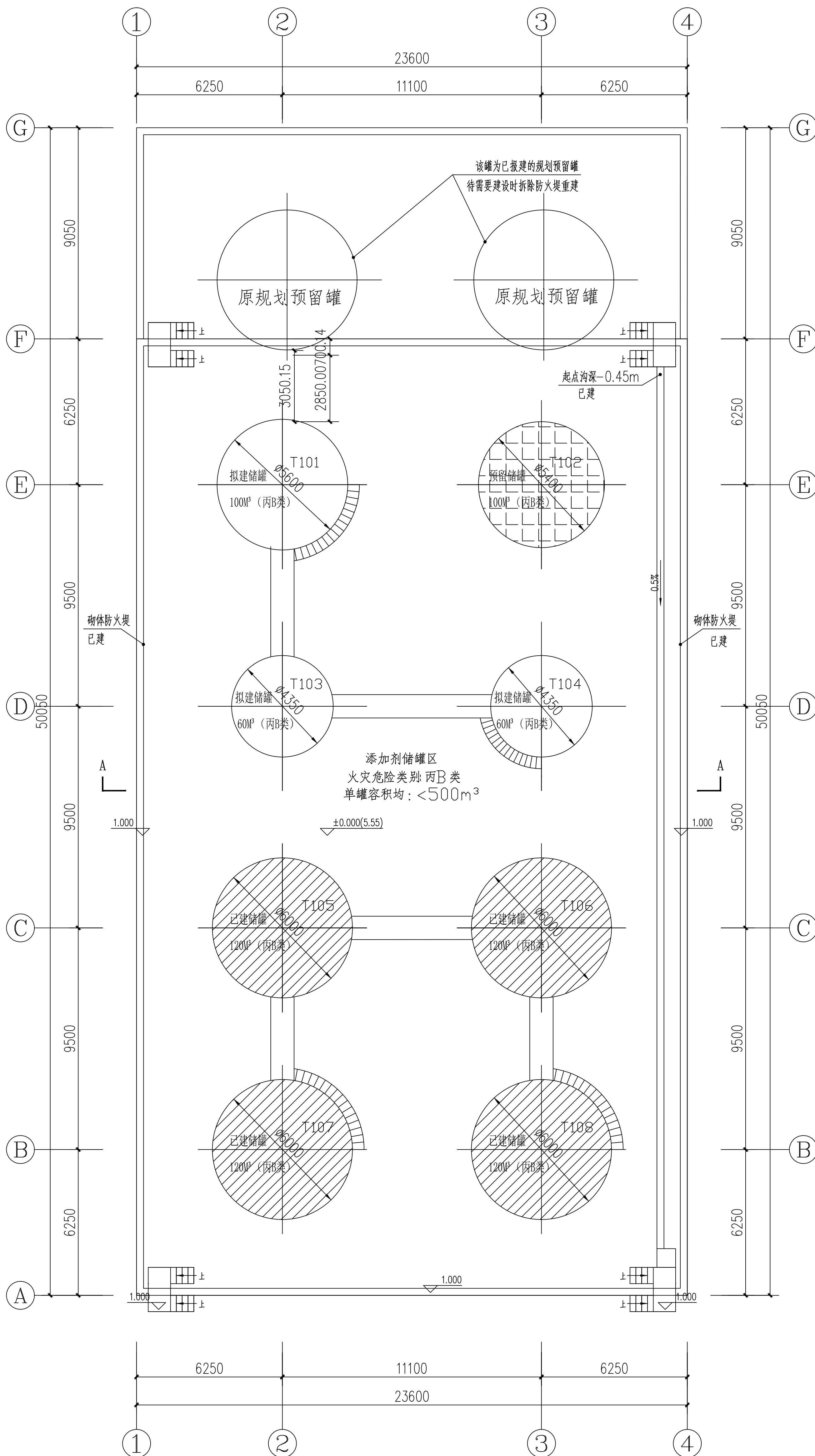
添加剂储罐区平面布置图
