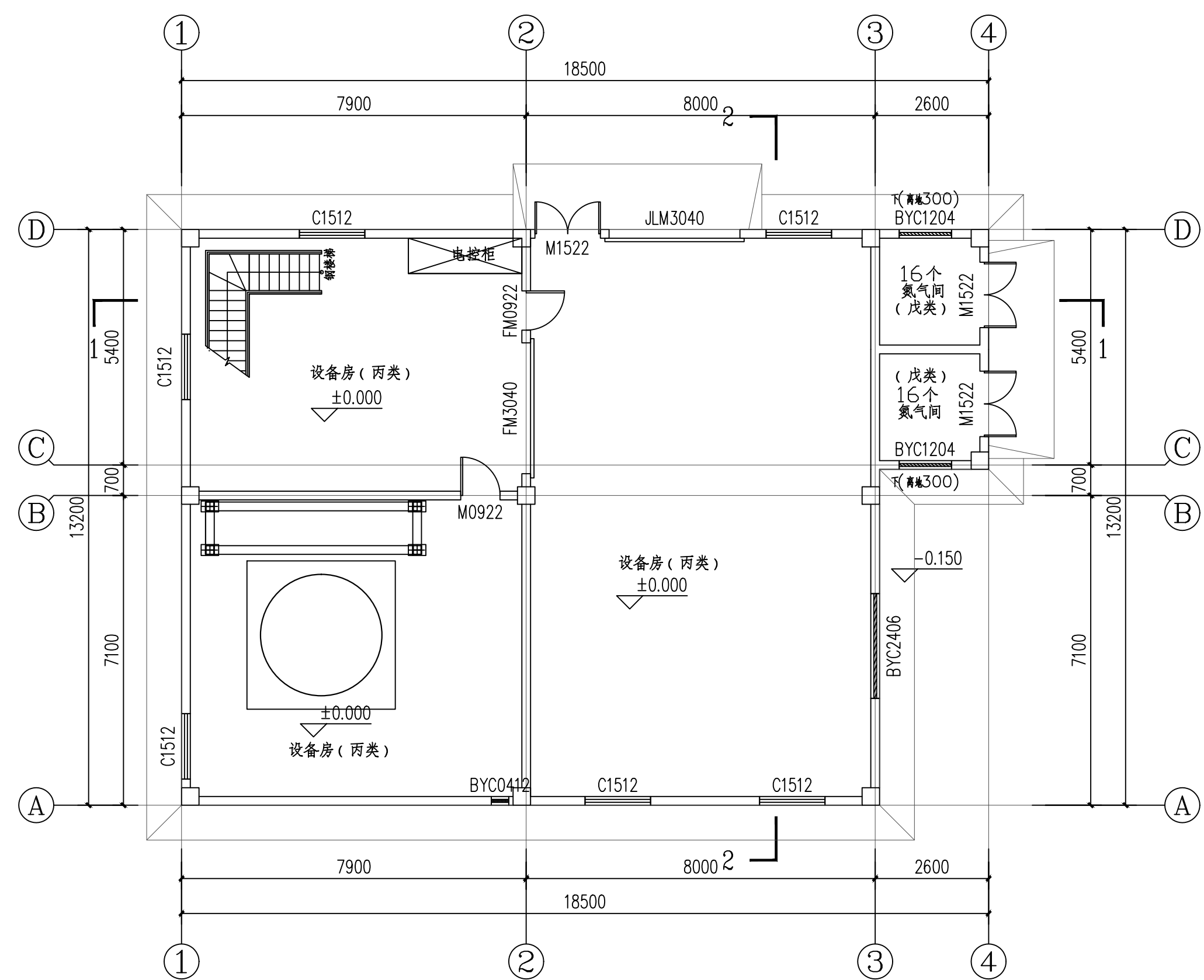
首层平面图
