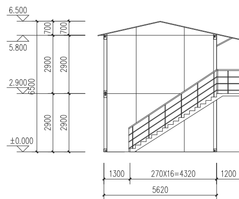
办公楼1左侧面立面图 1:100
