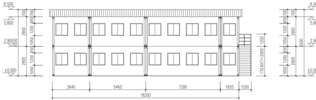
办公楼2背面立面图 1:100
