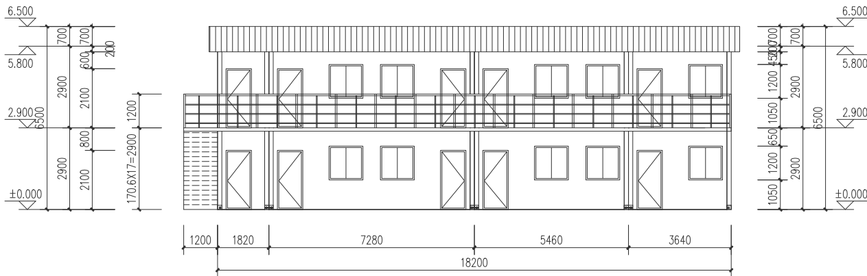
办公楼2正面立面图 1:100
