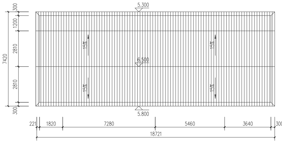
办公楼2屋顶层平面图 1:100
