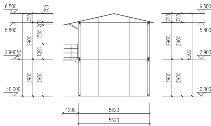
办公楼1右侧面立面图 1:100
