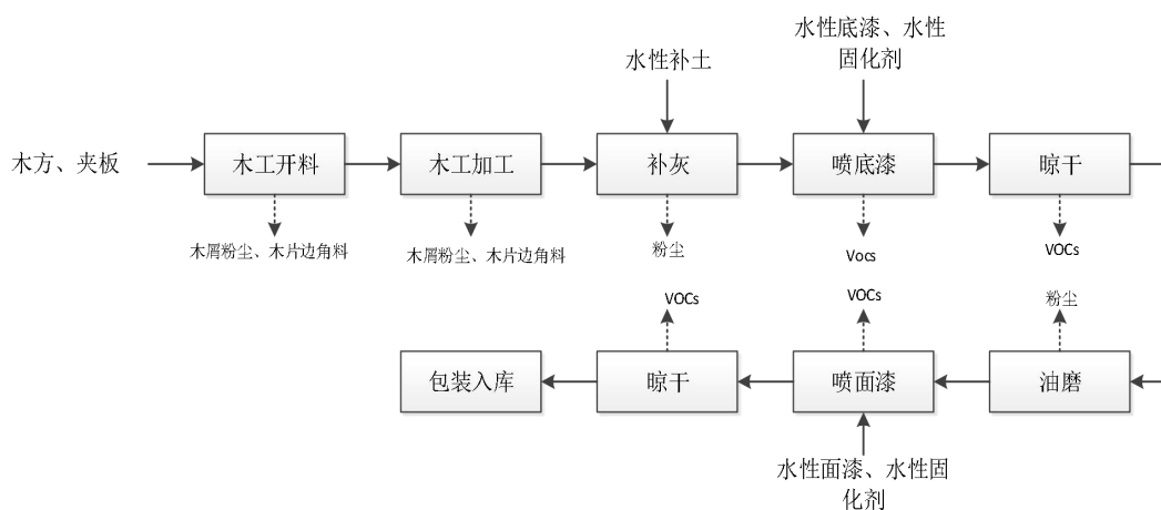
图 8 现有板式家具生产工艺流程图
