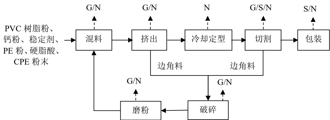
图6 木塑板家具生产工艺流程
