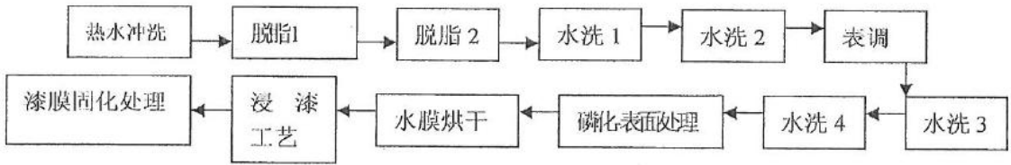
图 9 现有铁架生产工艺流程图
