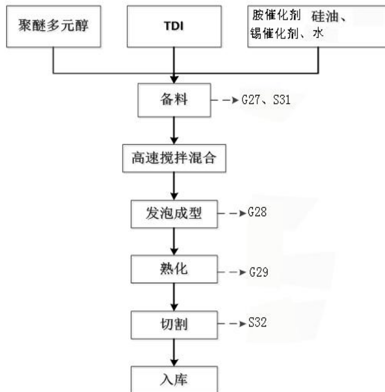
图 16 现有高密度海绵生产工艺流程图
