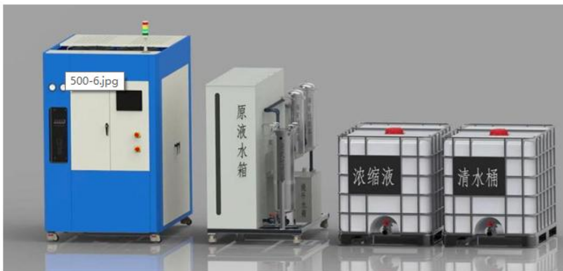
图 25 低温蒸发器示例设备图
