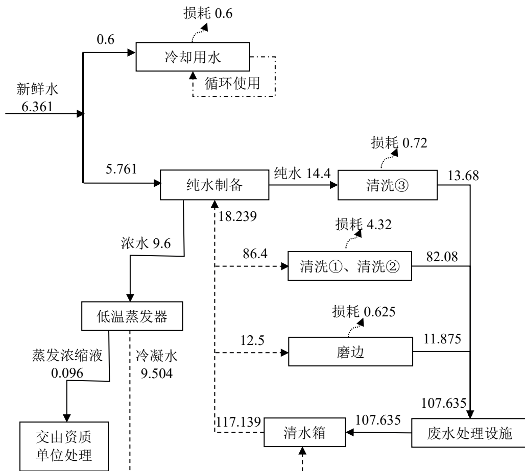
图 1 改扩建项目水平衡图 (t/d)
