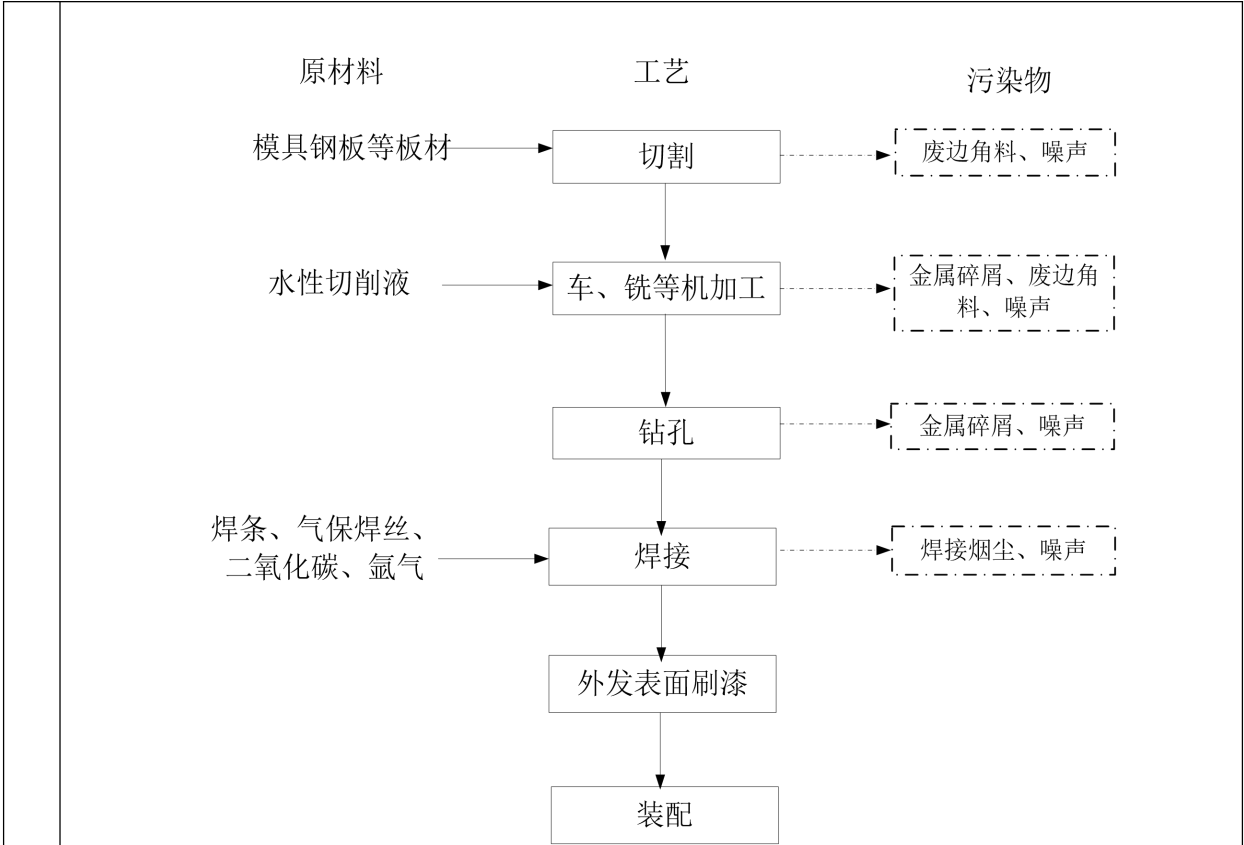
图 19 现有项目模具生产和维修工艺流程图及产污节点图
