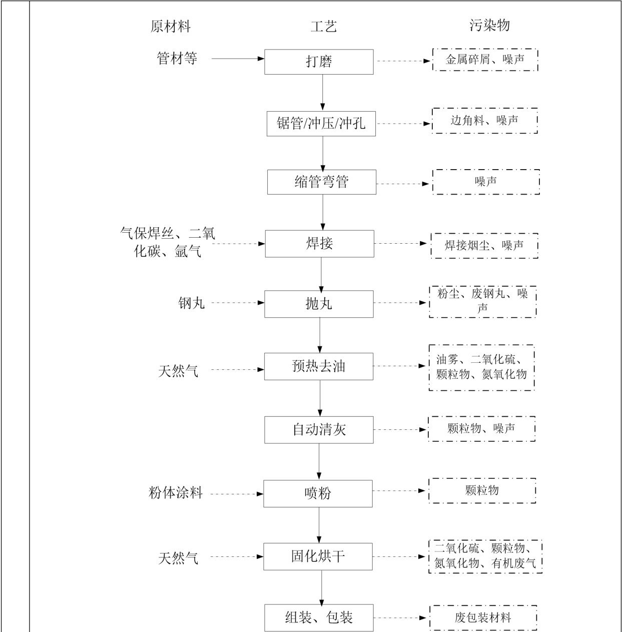
图 18 现有项目排骨架生产工艺流程图及产污节点图
