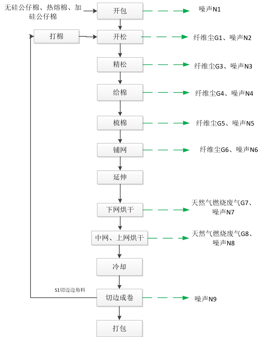
图 11 现有软绵生产工艺流程图
