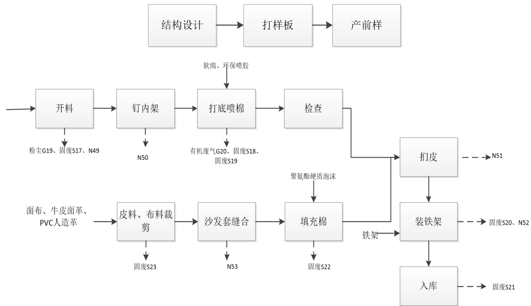
图 13 现有研发部沙发新产品生产工艺流程图
