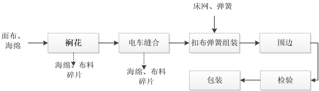
图 10 现有床垫生产工艺流程图
