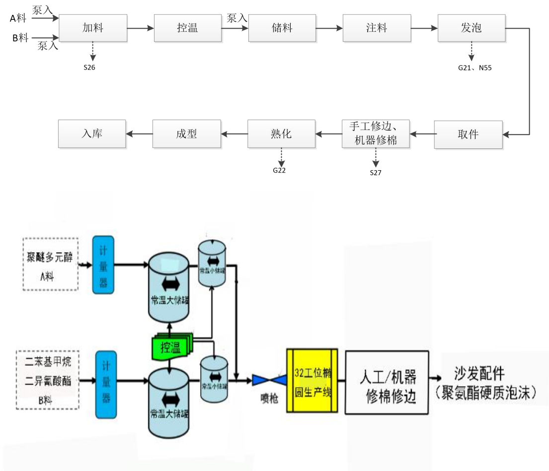
图 14 现有模具发泡生产工艺流程图
