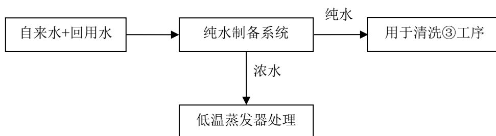
图 5 纯水制备流程图
