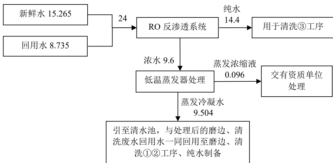
图 22 项目纯水制备过程示意图 (t/d)
