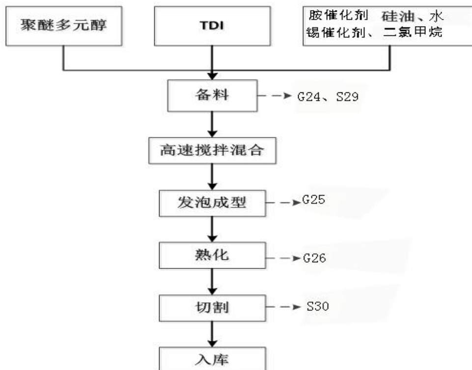
图 15 现有低密度海绵生产工艺流程图
