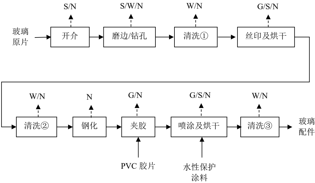
图3 玻璃配件生产工艺流程
