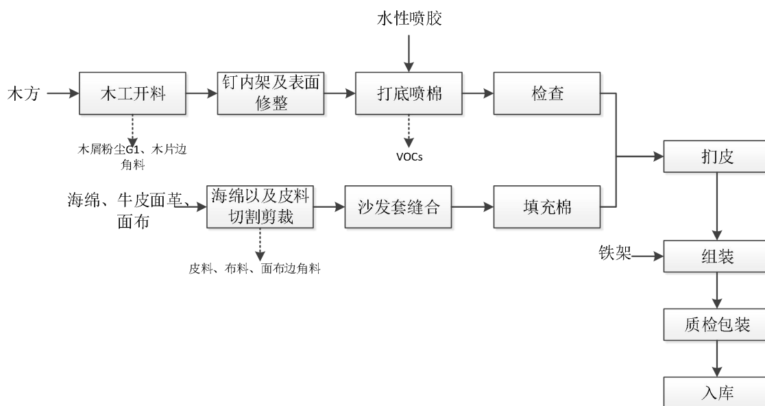
图 7 现有沙发生产工艺流程图
