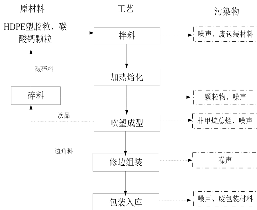
图 17 现有项目沙发塑胶部件生产工艺流程图及产污节点图
