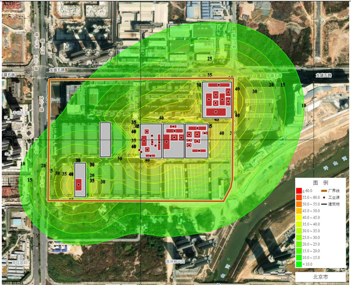
图23 改扩建项目噪声贡献预测等声级线图
