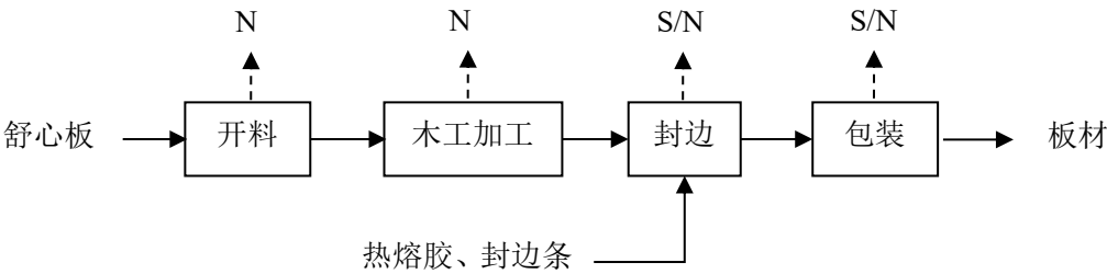
图2 板材生产工艺流程
