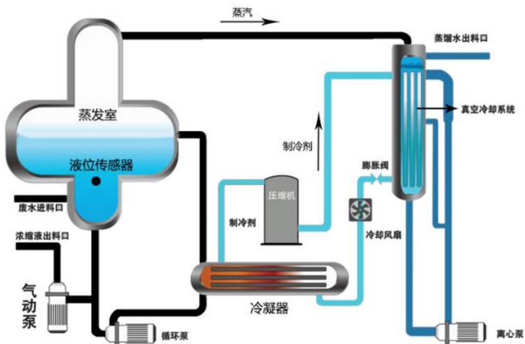
图 24 低温蒸发器工作原理示意图
