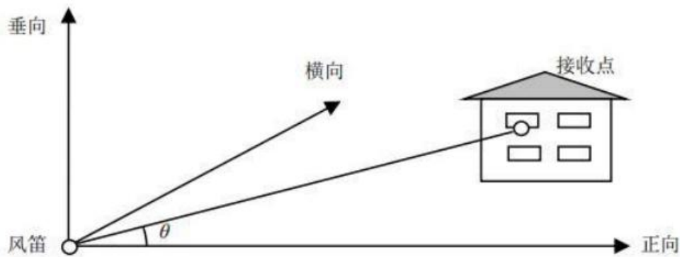
图 4-2 风笛指向性夹角θ示意图
